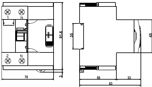
REC2 - 2 poles
