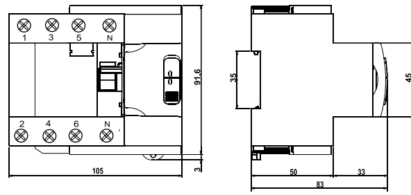
REC2 - 4 poles
